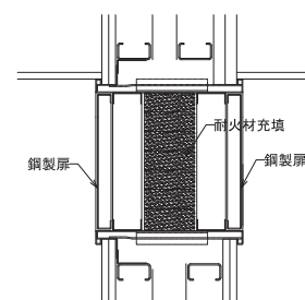
区画部貫通孔詳細
