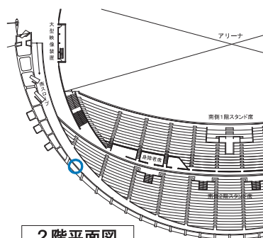
2階平面図
