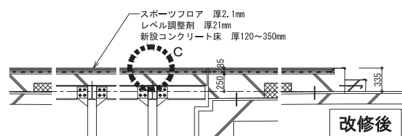
A-A断面図
