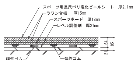
C部スポーツフロア詳細図
