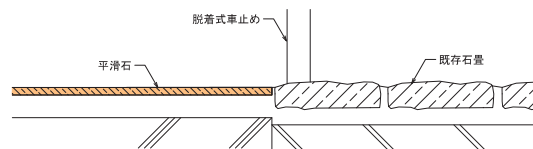
D-D断面図
