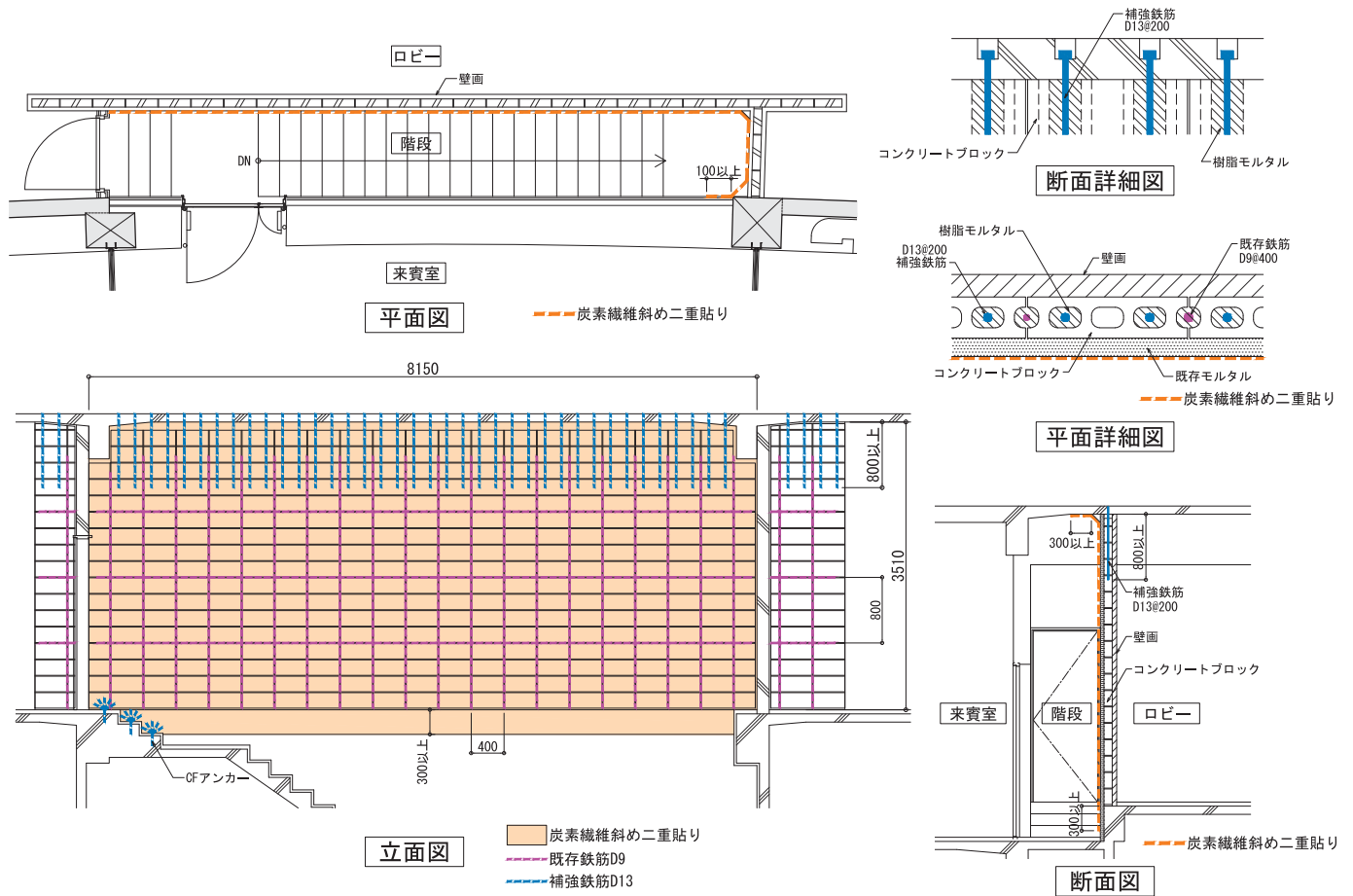
国立代々木競技場 第一体育館
