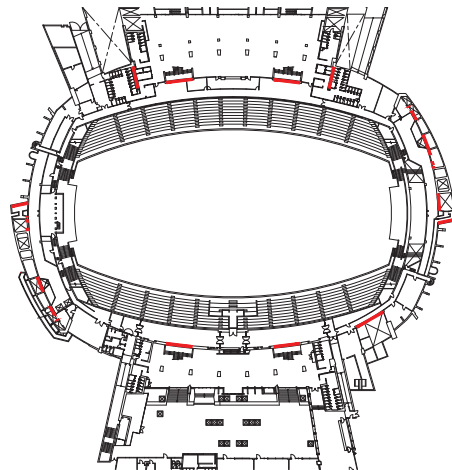
地下1階耐震補強範囲図
