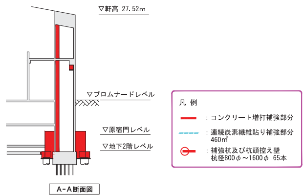
A-A断面図
