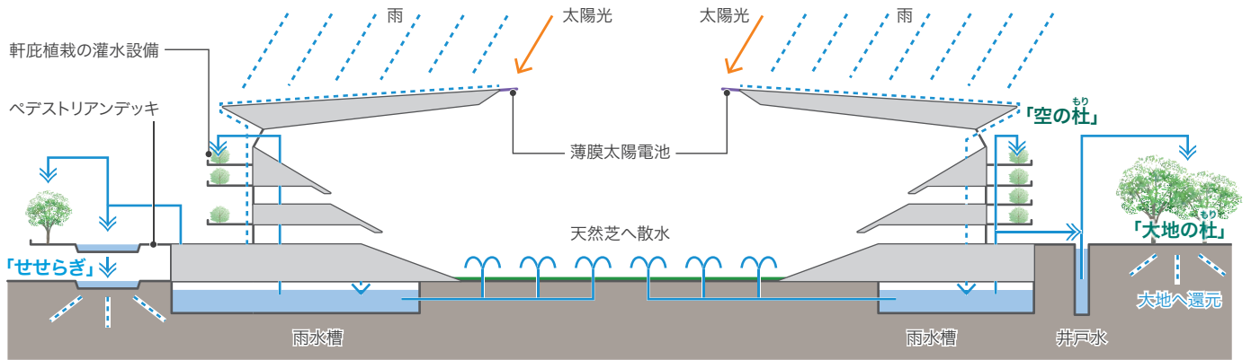
自然エネルギー利用イメージ
