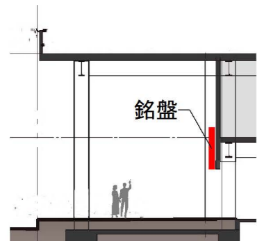
a-a断面 (銘盤配置イメージ)
