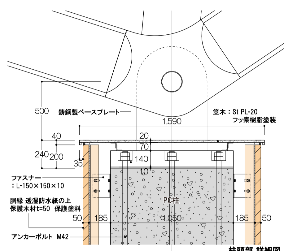
柱頭部 詳細図
