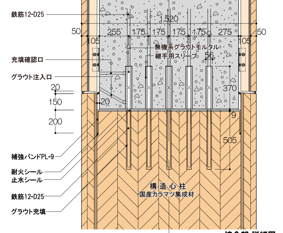
接合部 詳細図
