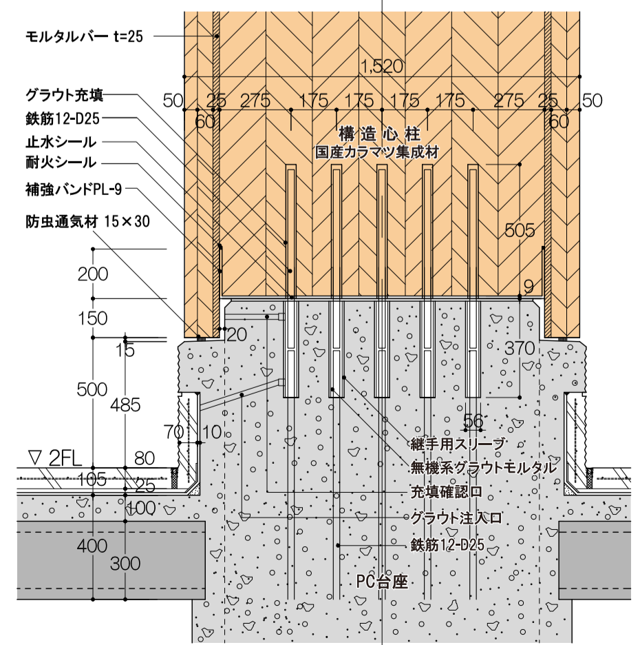
柱脚部 詳細図
