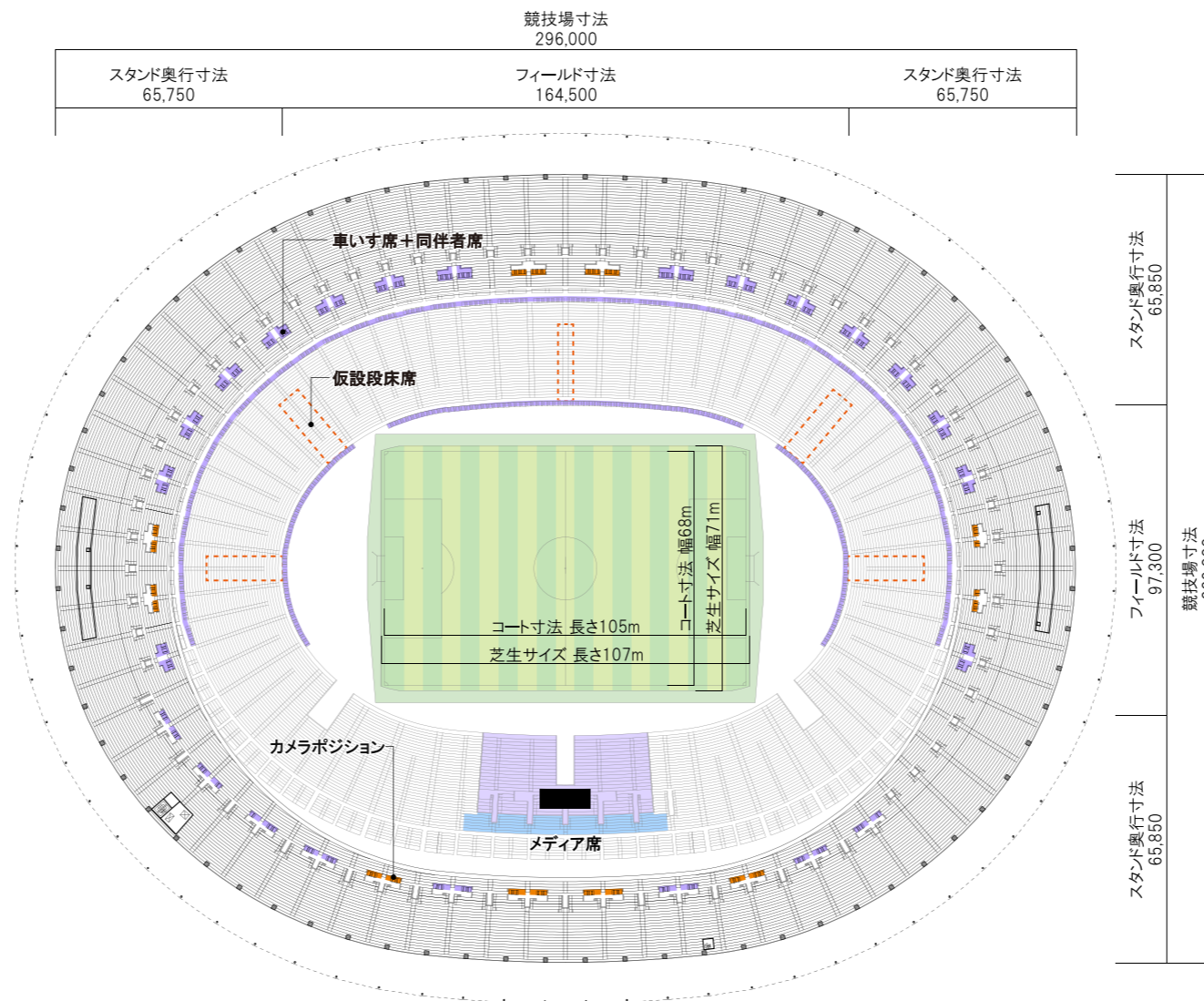
座席平面図 サッカー大会開催時(約80,000席)
