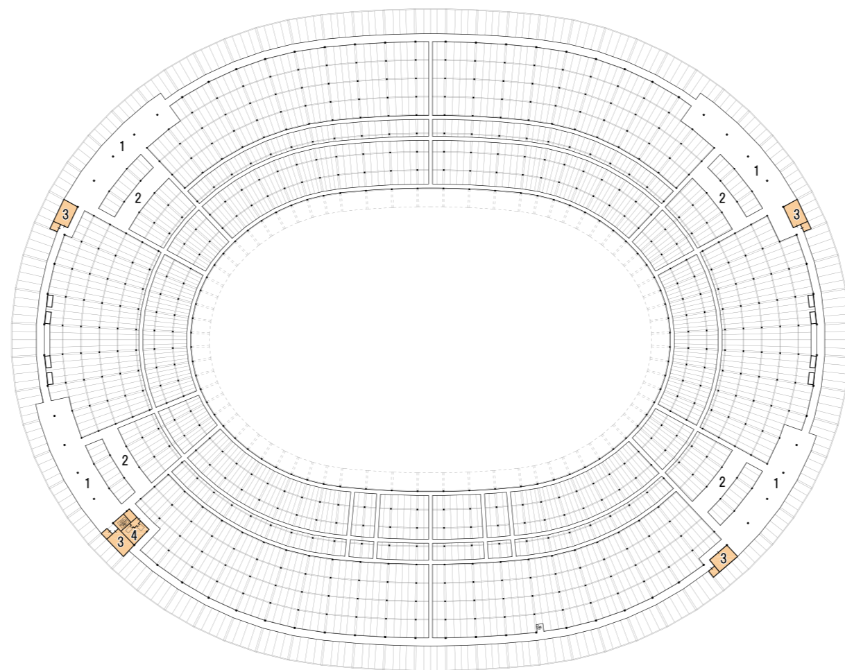
トラス階平面図
