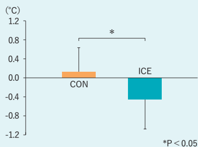
図2-15 脳温の変化
