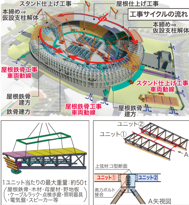
図⑤ 屋根部材ユニット化計画図 図⑥ 屋根鉄骨ユニット化接合部計画図
