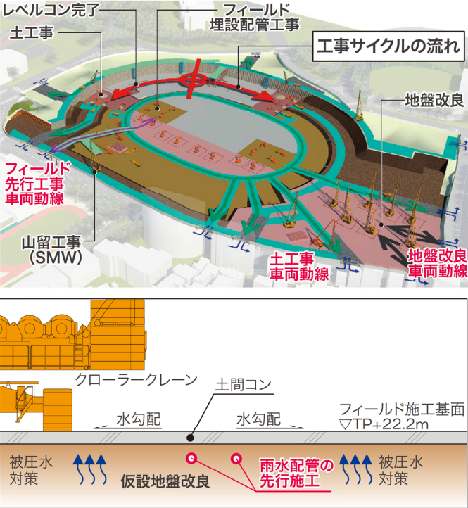
図① フィールド埋設配管・土間コンクリート計画図
