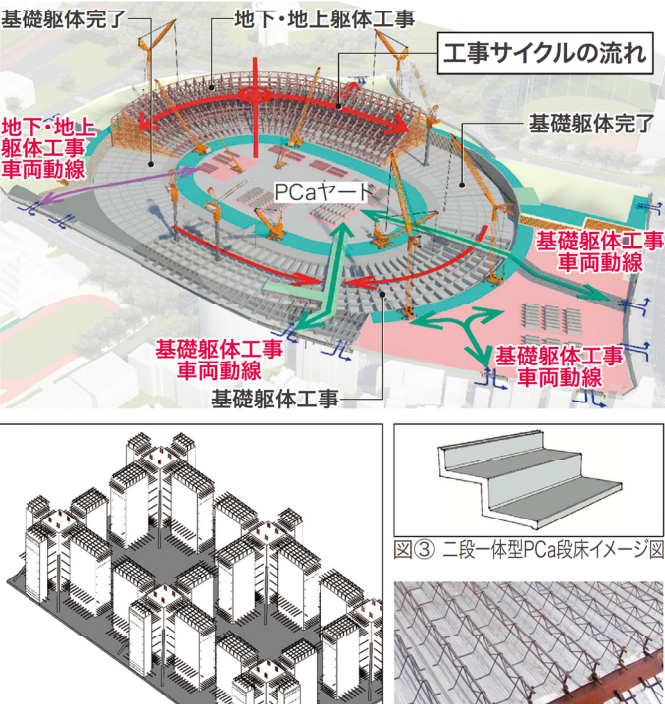
図② 基礎プレキャスト化計画図 図④ トラス筋付デッキイメージ
