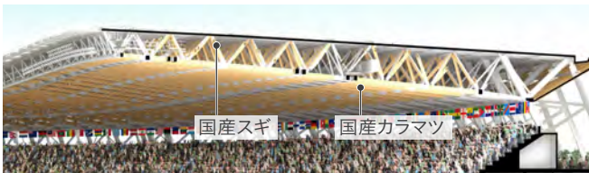
大屋根のトラスへの木材利用イメージ
